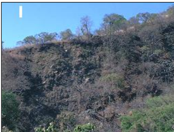
Foto 3, 4- Inestabilidades en la ladera sur 8 y 9 (izq), 10 (derch)
